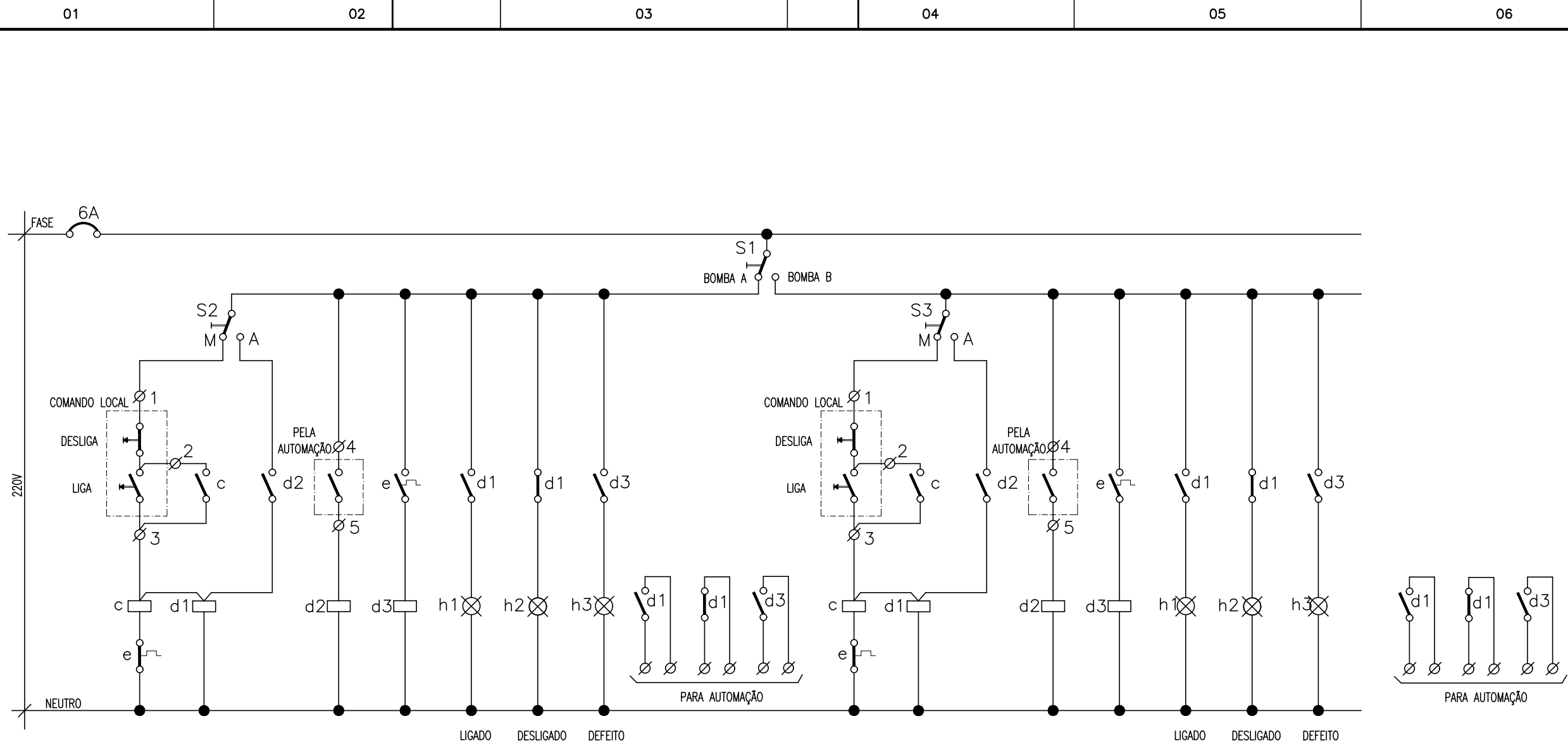
BOMBA BC-03A
