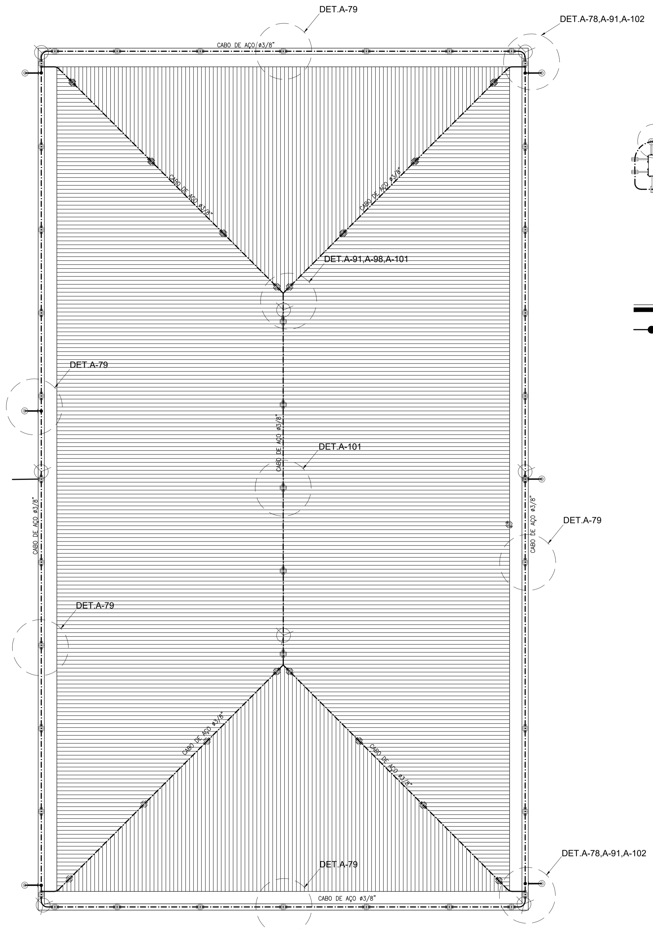
PRÉDIO DE APOIO PLANTA DE COBERTURA SPDA ESCALA 1:50
