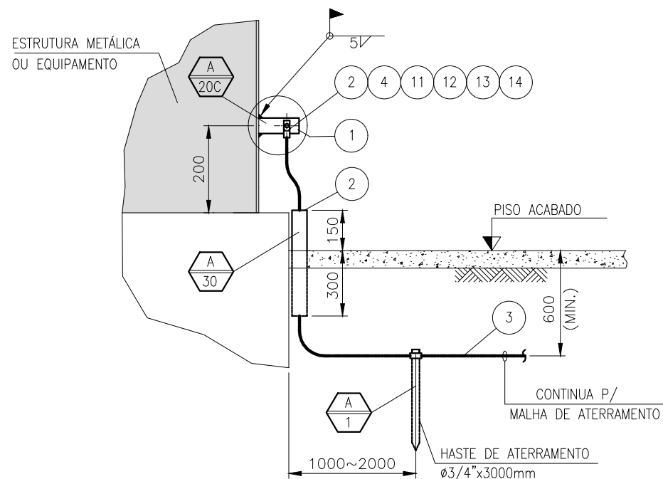
DETALHE A-9A PARA PROTEÇÃO ATMOSFÉRICA
