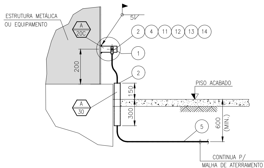
DETALHE A-9B PARA ATERRAMENTO DE CARGAS ELETROSTÁTICAS
